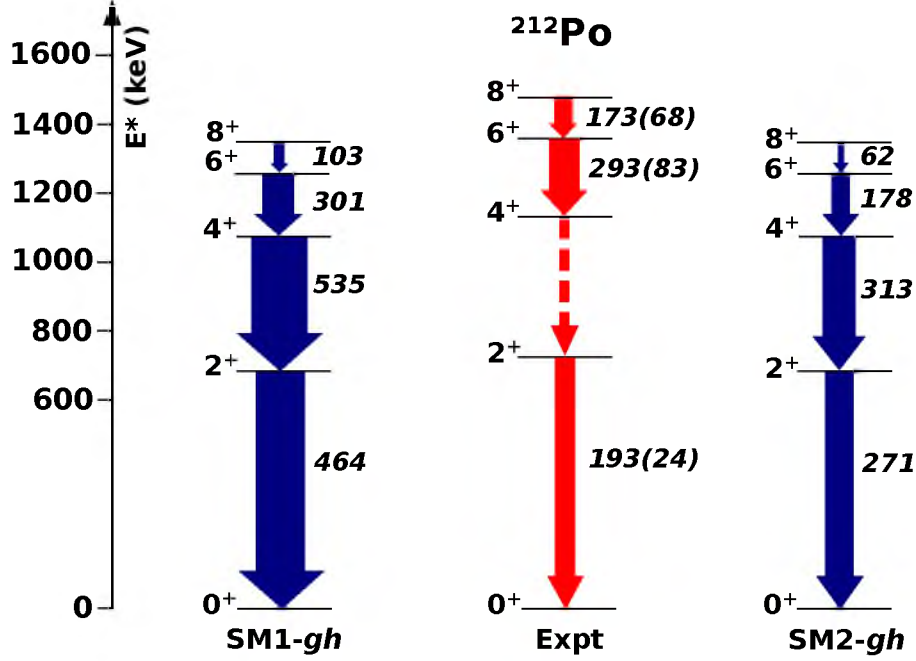
Фигура 8: Графично представяне на резултатите, получени в рамките на слоестия модел в едноконфигурационно приближение ( SM1-gh и SM2-gh ) за състоянията от основната ивица в ^{212}\text{Po} , сравнени с експериментално определените такива ( Expt ). Дебелината на стрелките е пропорционална на B(E2; 2_1^+ \rightarrow 0_1^+) стойностите, които са представени до стрелките в единици \text{e}^2\text{fm}^4 .
