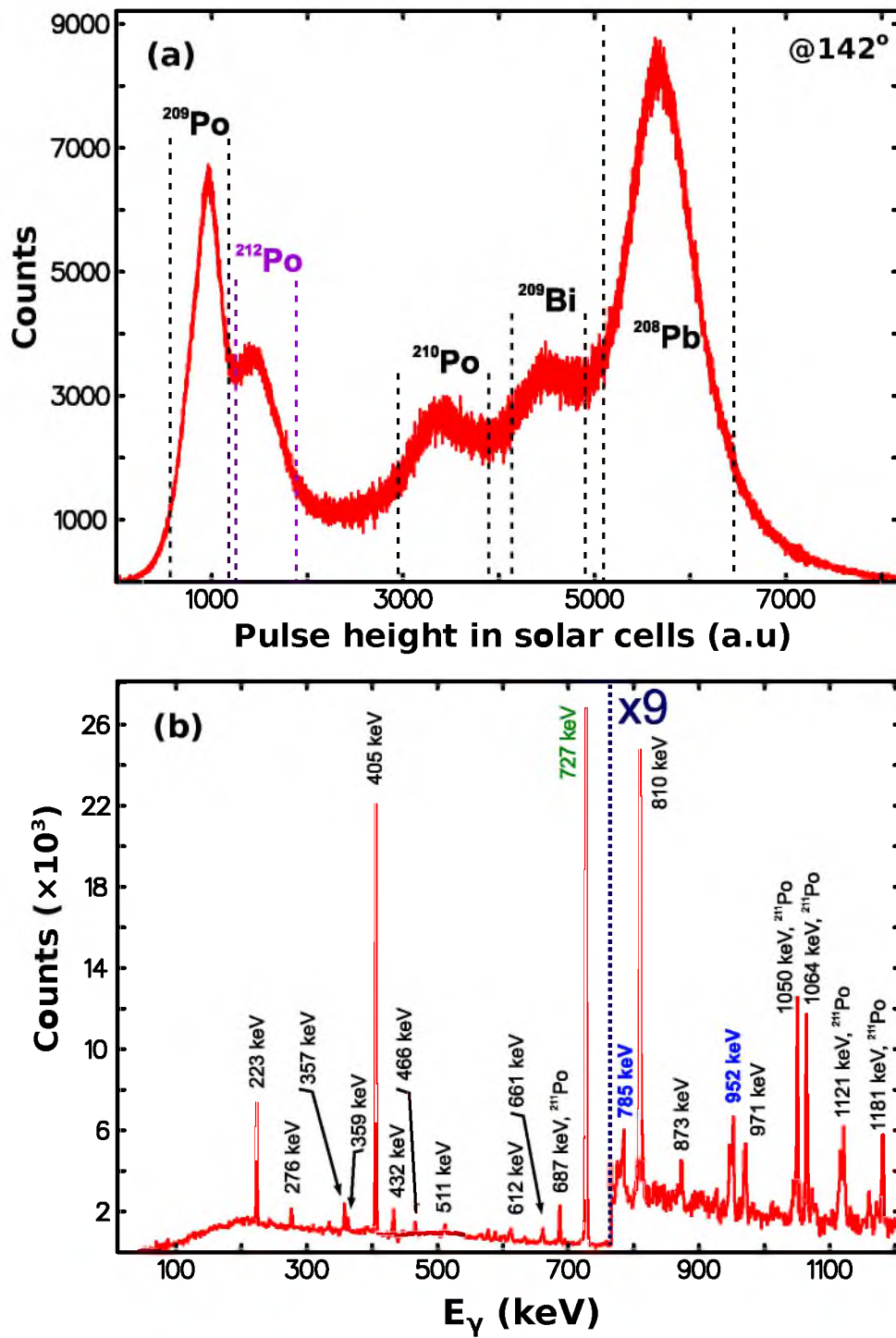
Фигура 2: (а) Проекция на матрицата на съвпадение между частици и \gamma -кванти на 142^\circ . Заградените области представляват частици, които са в съвпадение с \gamma -лъчи от съответните ядра. (b) Спектърът на \gamma -лъчи, получен в съвпадение с частта на частици, обозначени като " ^{212}\text{Po} " в (а).
