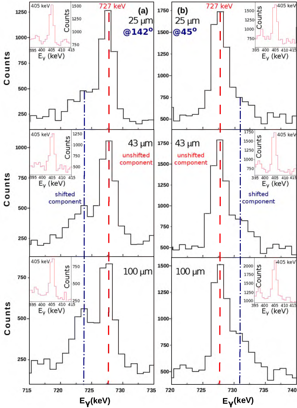
Фигура 5: Отместените и неотместени компоненти на линията с енергия 727 keV ( 2_1^+ \rightarrow 0_1^+ ) на задни (a) и предни ъгли (b) за три различни разстояния между мишената и стопера: 25 μm, 43 μm, 100 μm. В горните ъгли е показана линията на прехода с енергия 405 keV ( 4_1^+ \rightarrow 2_1^+ ) за съответните ъгли и разстояния.
