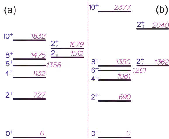
Фигура 7: Сравнение между експериментално наблюдаваните нисколежащи възбудени състояния в ядрото ^{212}\text{Po} (a) с теоретично пресметнатите (b). Енергиите на нивата са дадени в keV.
